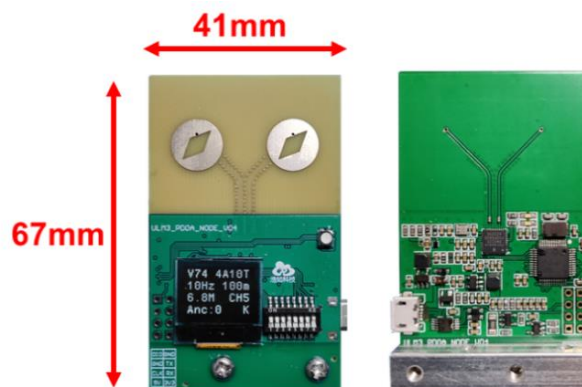
图 3-1 ULM3-PDOA 模块外观图
