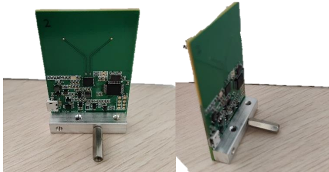
图 6-3 底部固定块增加铜柱支撑
