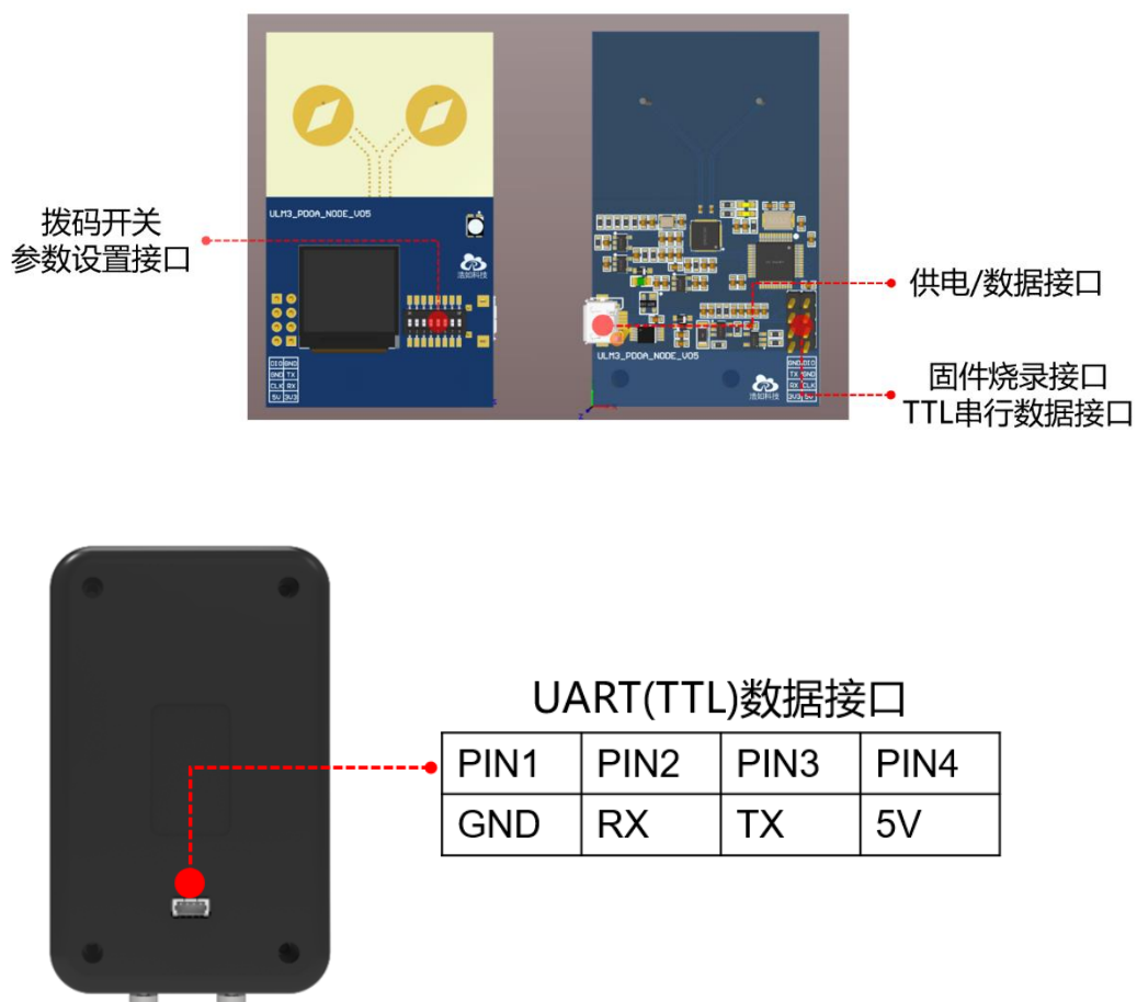
图 5-1 模块接口
