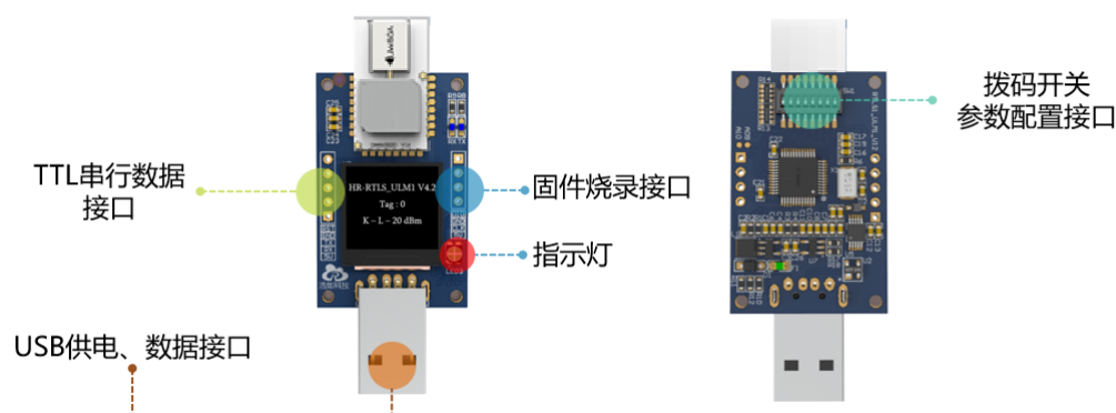
图 5-1 模块接口
