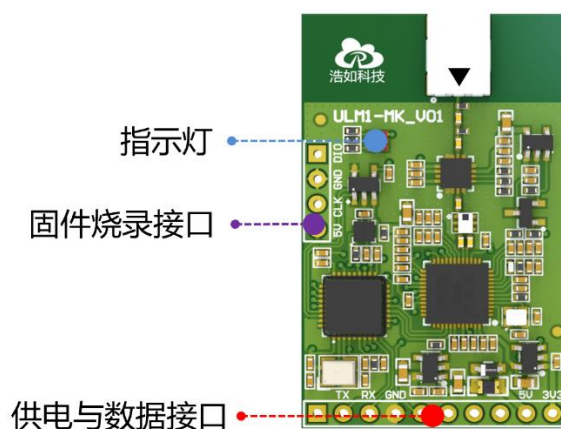
图 4-1 模块接口示意图
