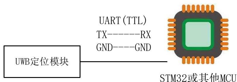
图 4-2 模块 TTL 串行数据接口示意图
