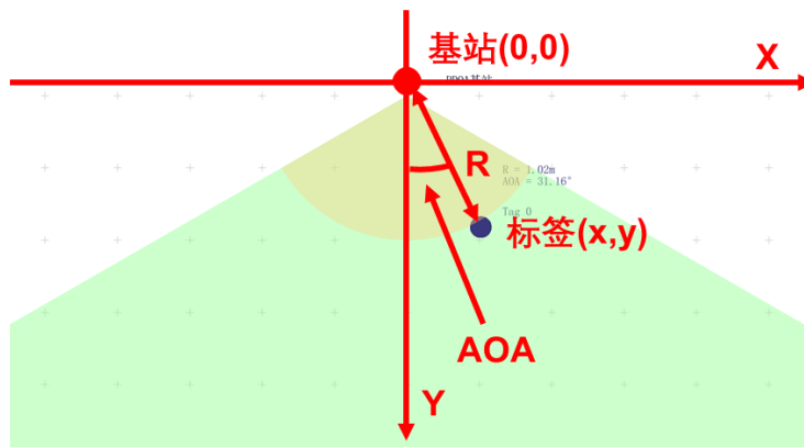
图 6-3 定位范围和坐标系
